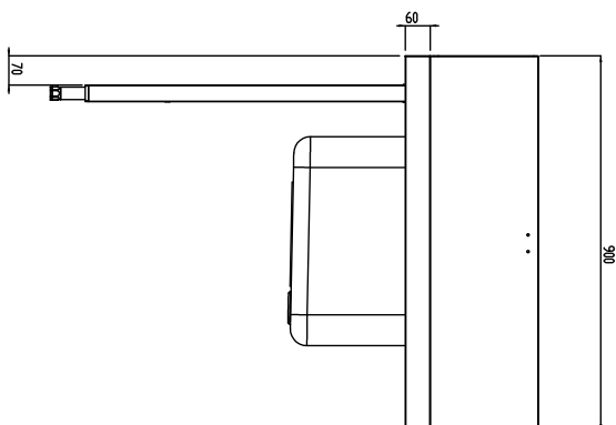
Zij aanzicht
