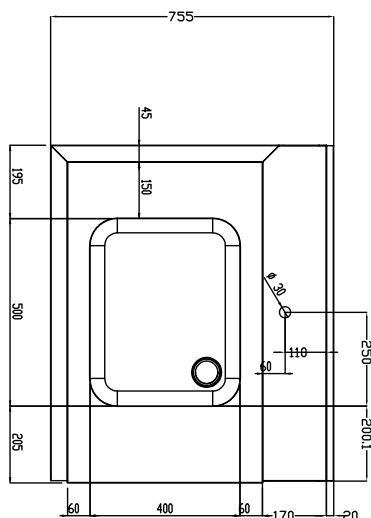
Boven aanzicht
